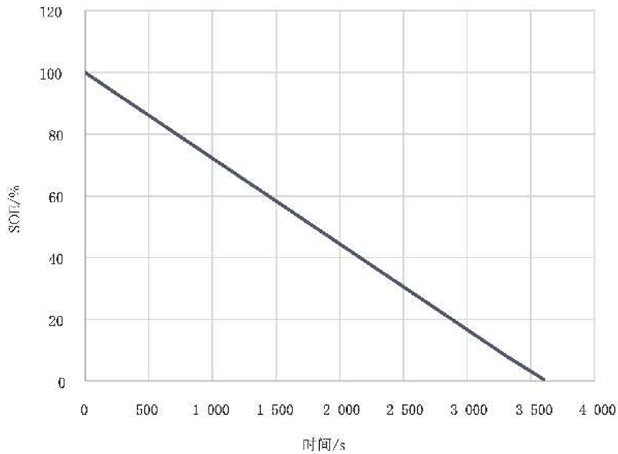
图 D.4 电池放电 SOE-时间曲线
