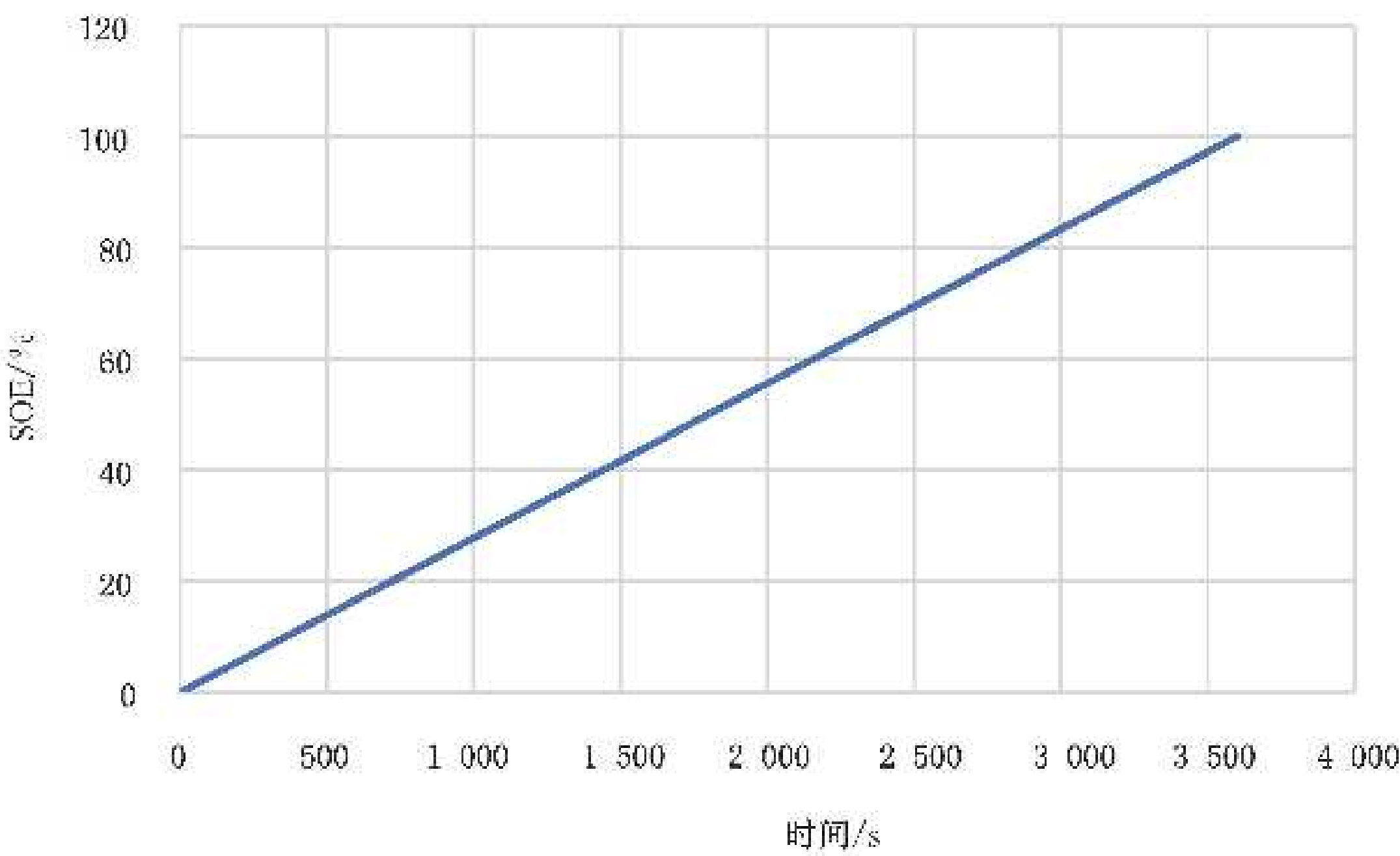
图 D.2 电池充电 SOE-时间曲线
